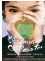
Mecánicas celestes
